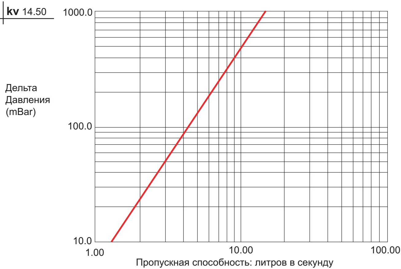
Диаграмма 990844/TA/3: зависимость падения загрузки от пропускной способности магнитного противоиловного аппарата ELCLA5 Ø 2".
