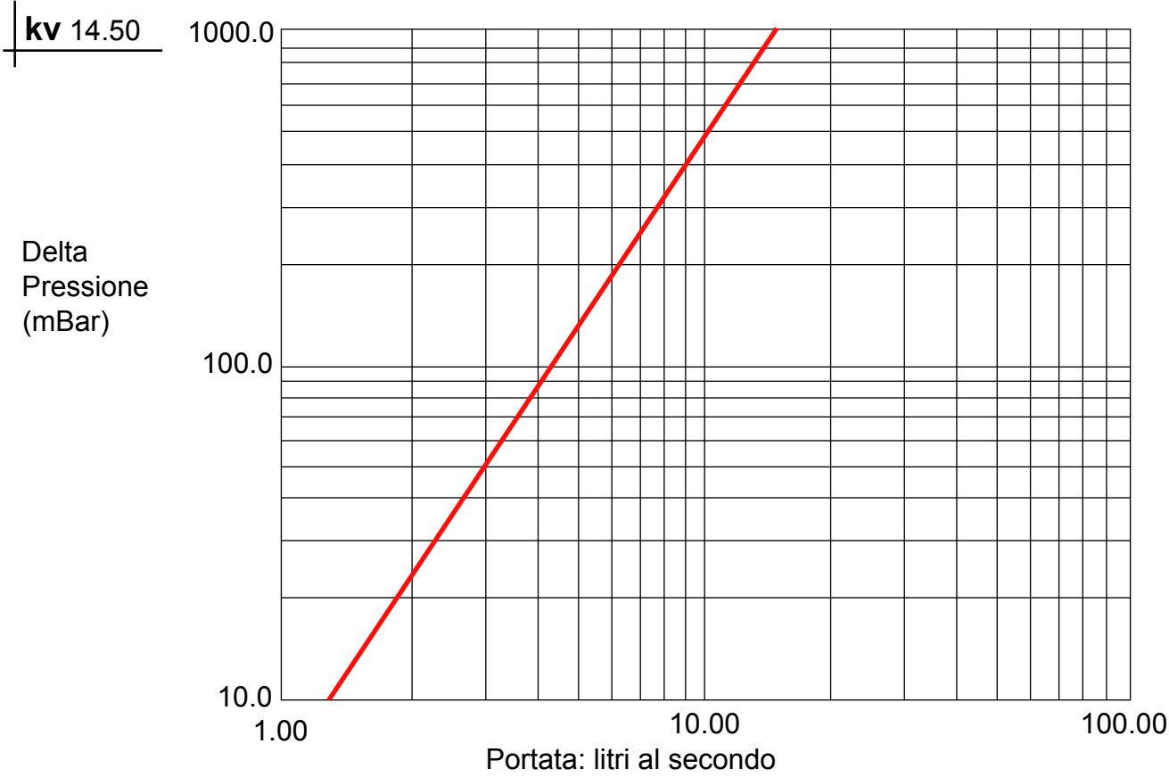
Diagramma 990844/TA/3: determinazione della perdita di carico contro portata dell'anticalcare magnetico ELCLA5 Ø 2".
