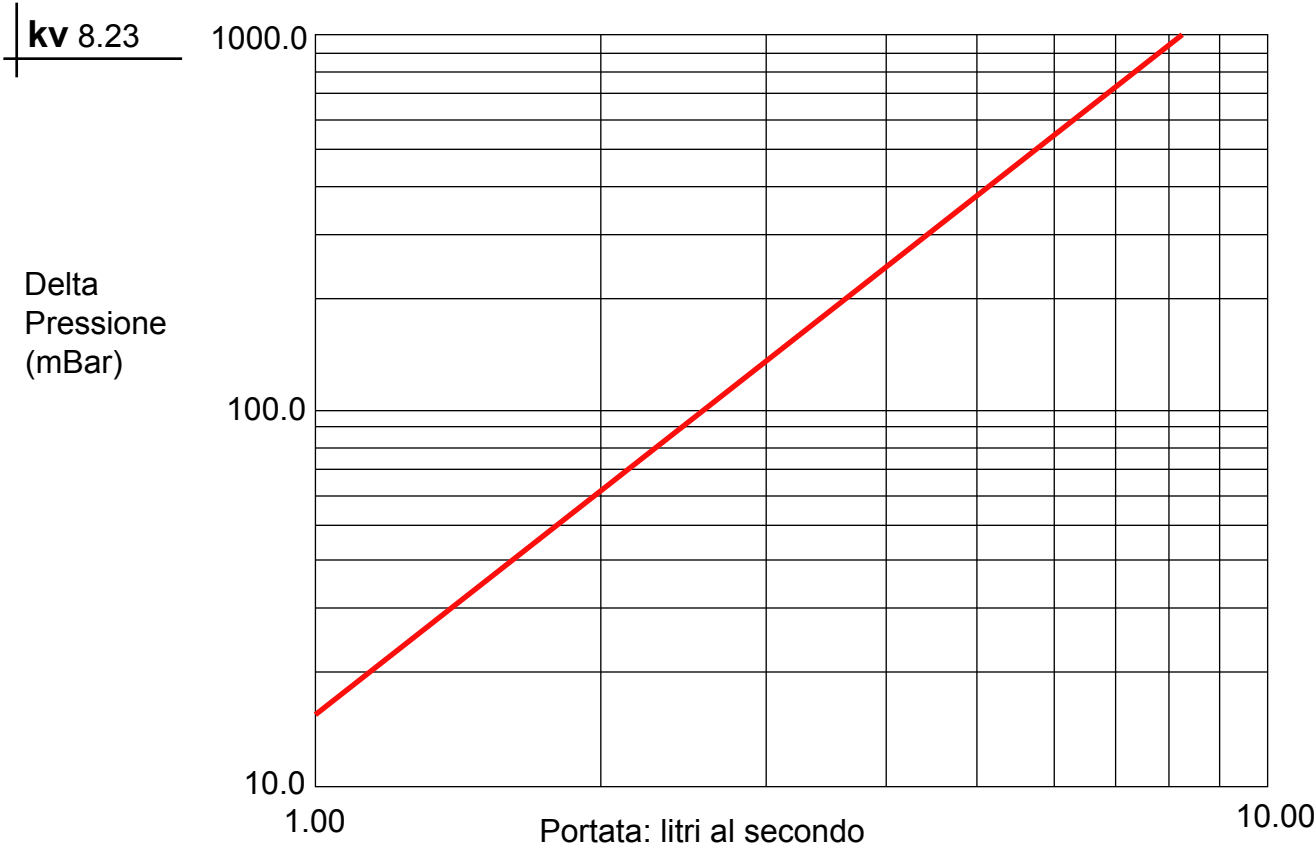
Diagramma 990844/TA/2: determinazione della perdita di carico contro portata dell'anticalcare magnetico ELCLA4A Ø 1.1/2".
