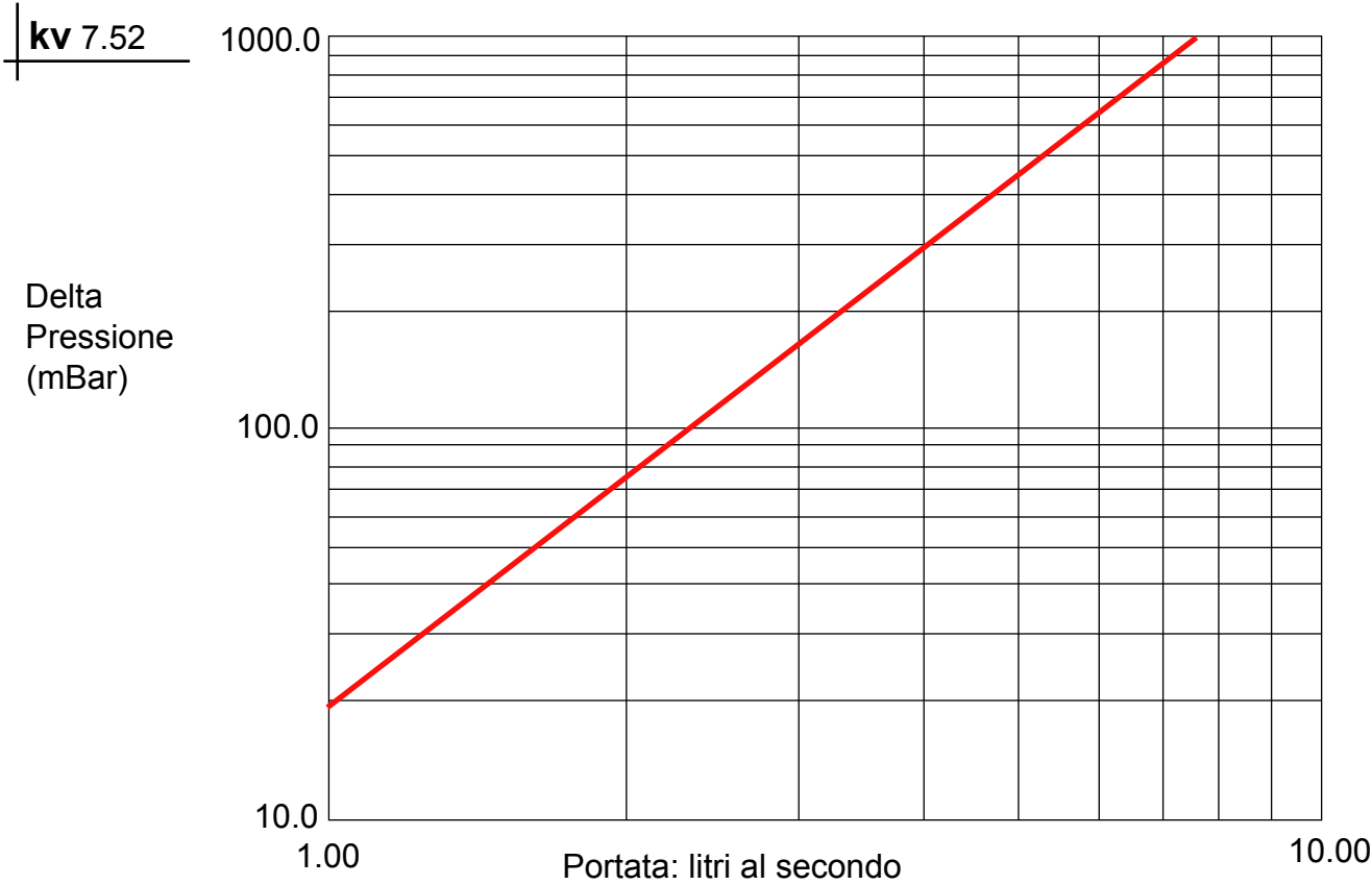
Diagramma 990844/TA/1: determinazione della perdita di carico contro portata dell'anticalcare magnetico ELCLA4 Ø 1.1/4".
