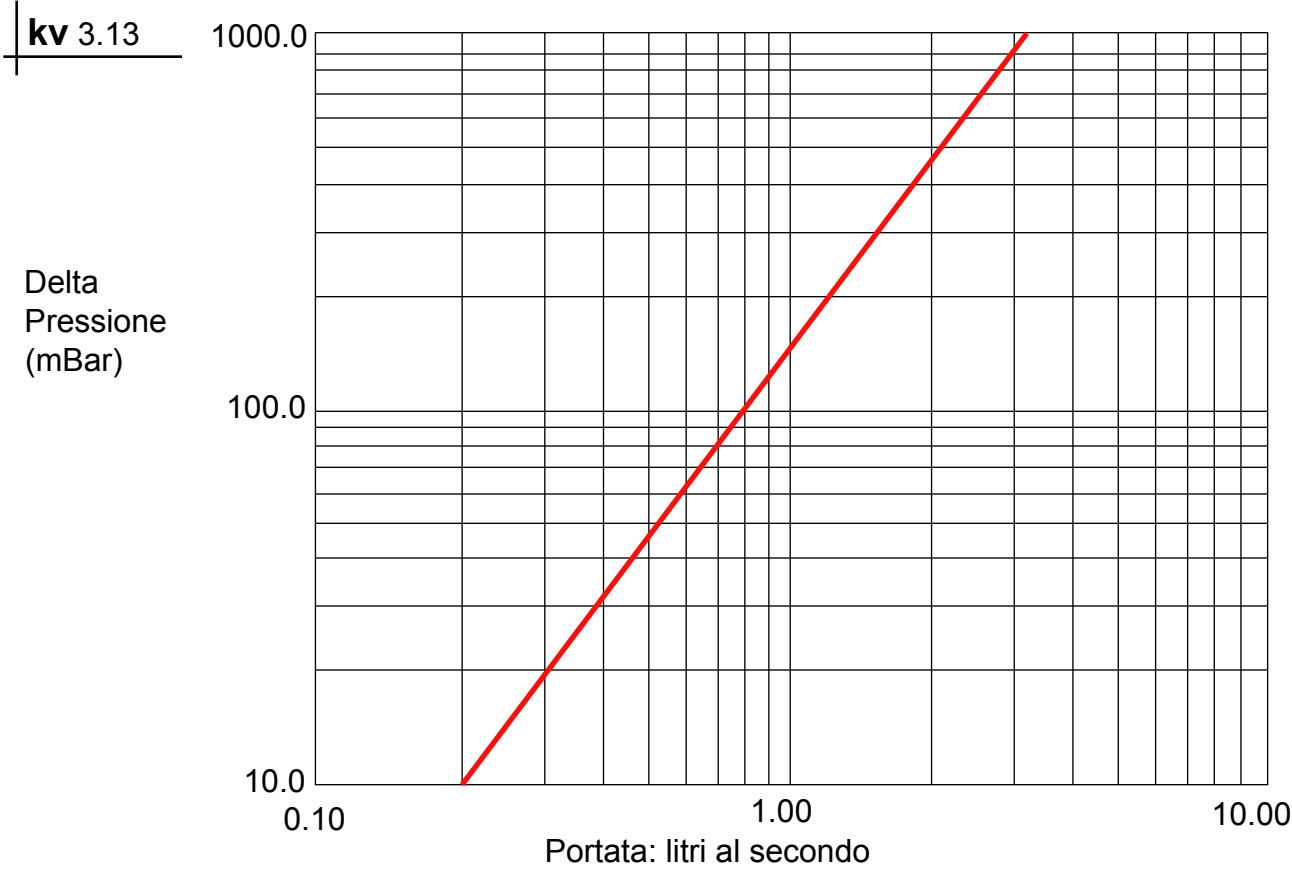
Diagramma 981559/4: determinazione della perdita di carico contro portata dell'anticalcare magnetico ELCLA3 Ø 1".
