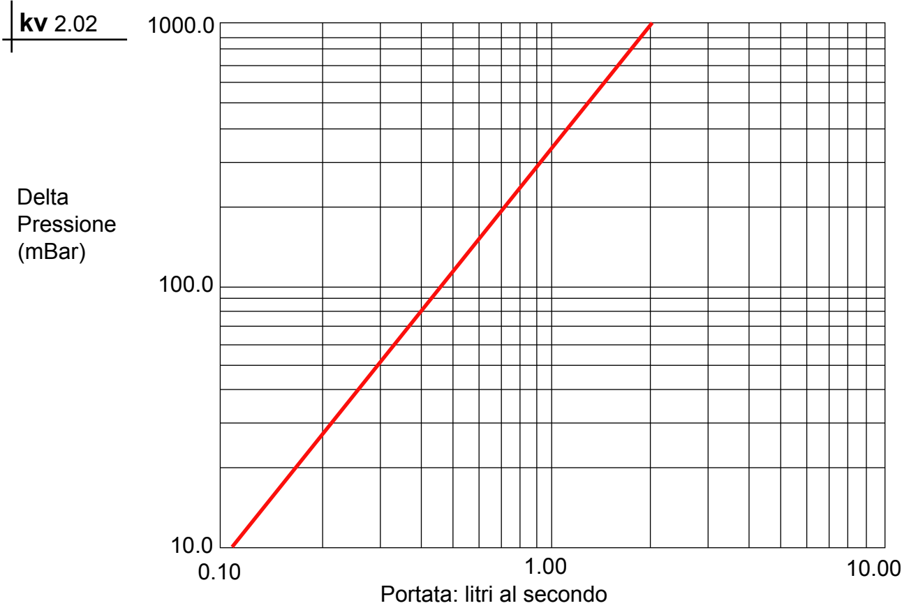
Diagramma 981559/2: determinazione della perdita di carico contro portata dell'anticalcare magnetico ELCLA1 Ø 1/2".
