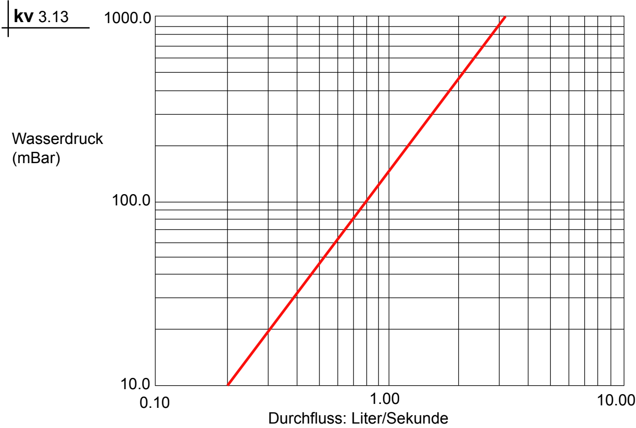
Diagramm 981559/4: Angabe vom Druckverlust durch den magnetischen Entkalker ELCLA3 Ø 1".
