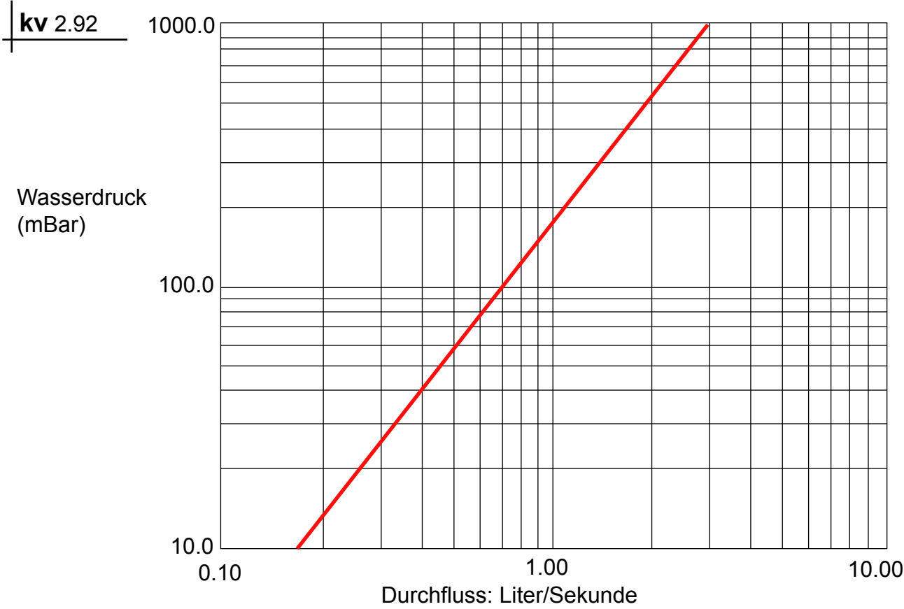
Diagramm 981559/3: Angabe vom Druckverlust durch den magnetischen Entkalker ELCLA2 Ø 3/4".
